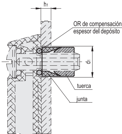
4.7 < h_1 < 6.3 (montaje con junta tórica)
