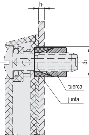
1.5 < h_1 < 4.7 (montaje sin junta tórica)
